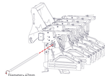
sześciokątny wał przekładni-42 mm
